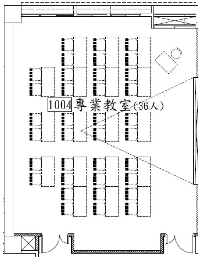
平面圖
